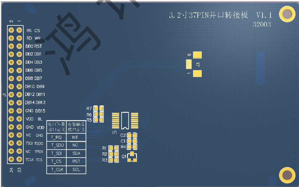
背面图
